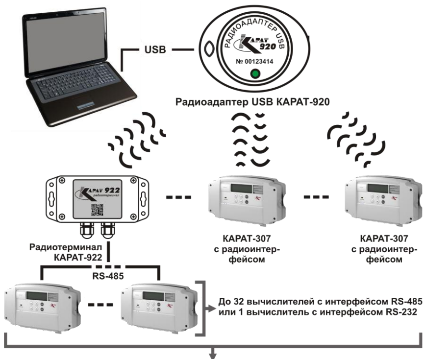
Рисунок В.7 – Принципиальная схема передачи данных по радиointерфейсу с использованием радиоадаптера USB KARAT-920 и радиотерминала KARAT-922
