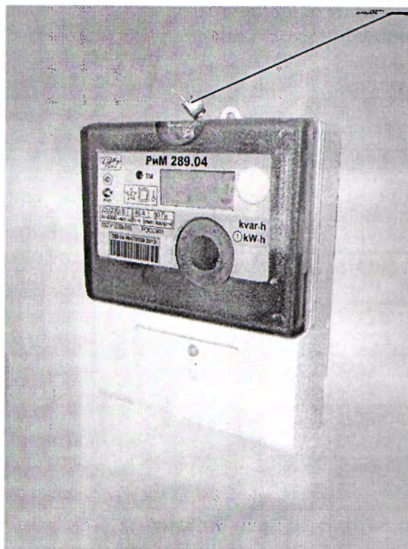
Рисунок 2 – Фотография общего вида и место установки пломбы поверителя счетчиков РиМ 289.04
