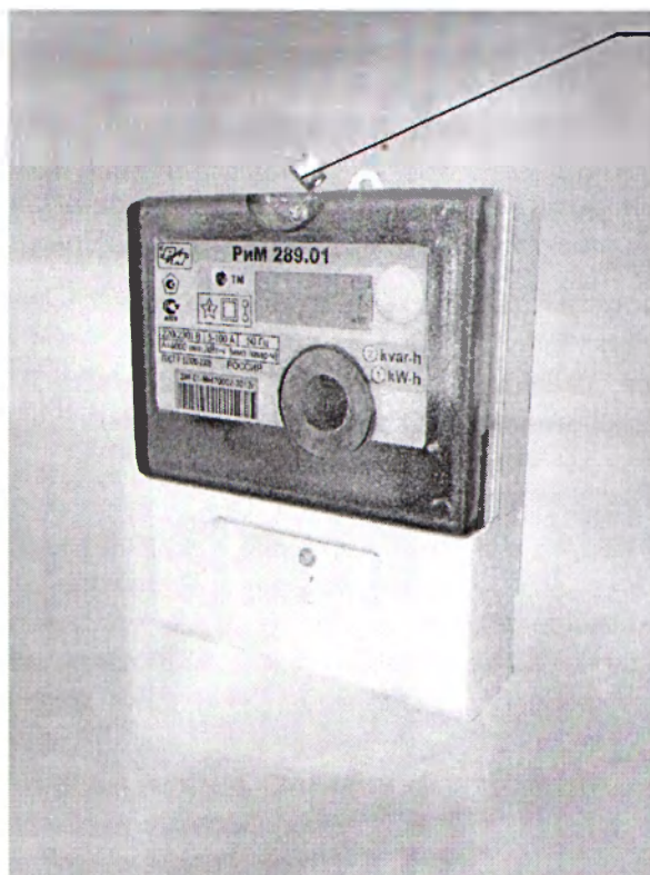
Рисунок 1 – Фотография общего вида и место установки пломбы поверителя счетчиков РиМ 289.01
